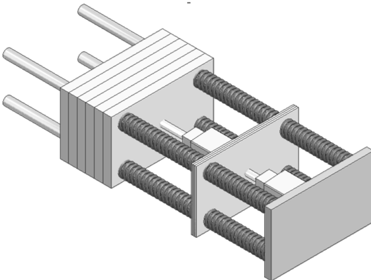
Figura 5 - Desenho em 3D da suspensão em conjunto
