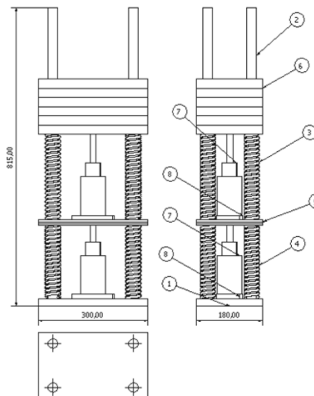
Figura 4 - Conjunto do Sistema de Amortecimento
