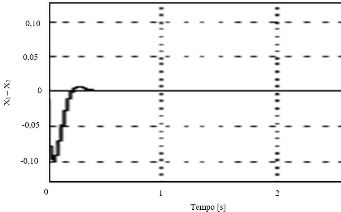
Figura 6 - Resposta em MF (Malha Fechada) a uma perturbação degrau de 15 cm
